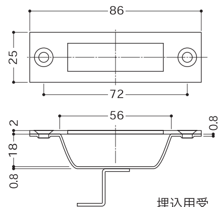
埋込用受
