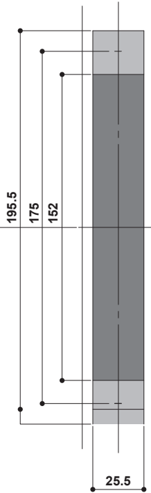
ドア切欠図
