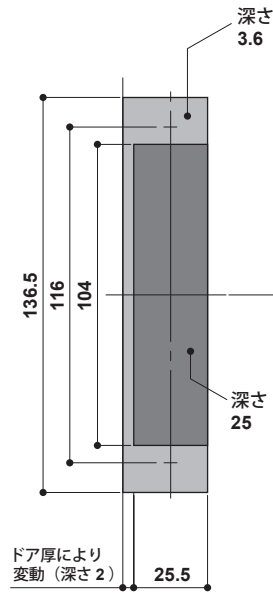
ストライク切欠図
