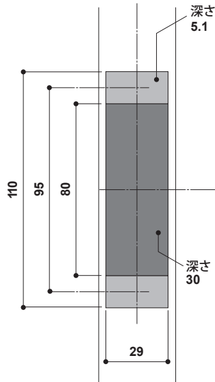
ストライク切欠図
