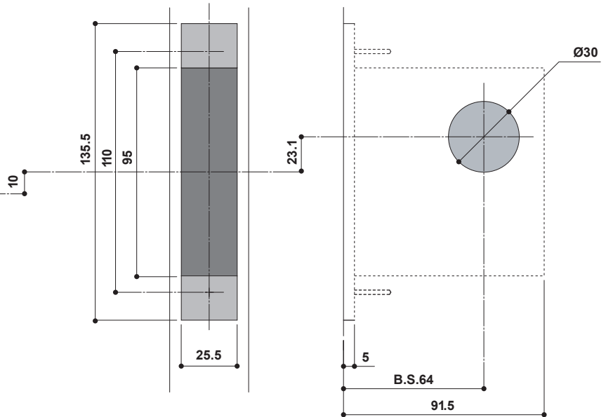
ドア切欠図
