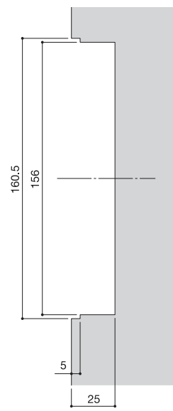
434プレートタイプ切欠図
