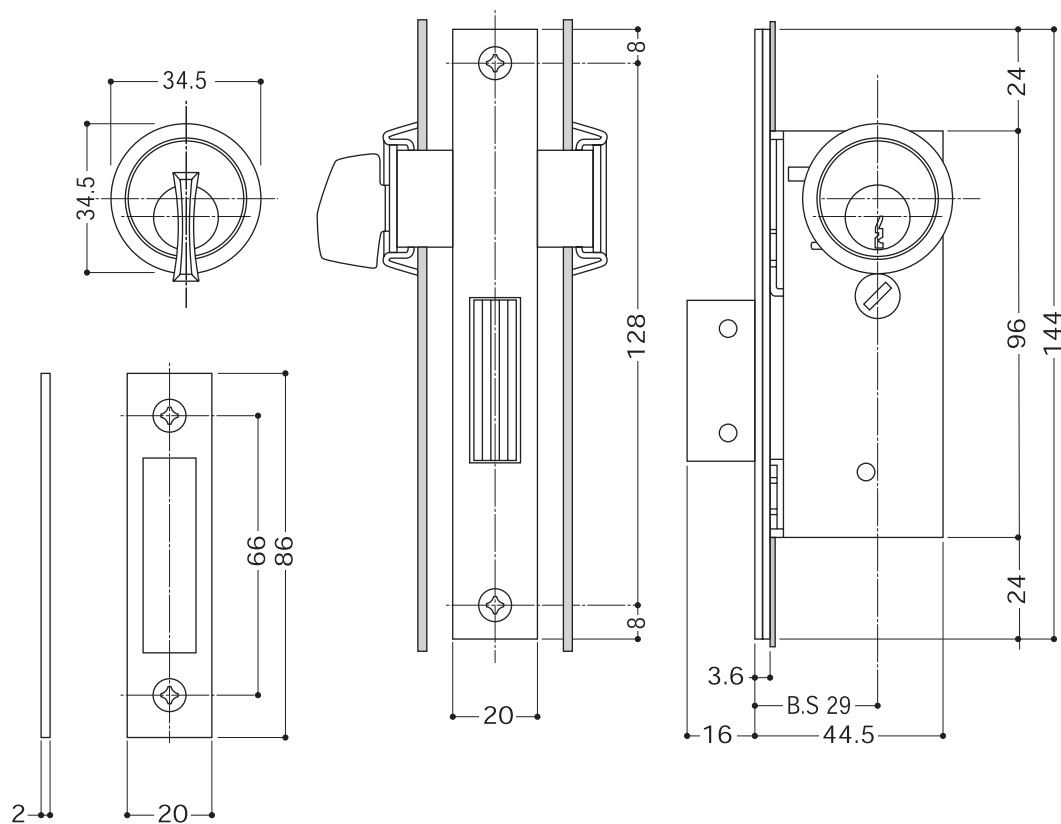
詳細図
